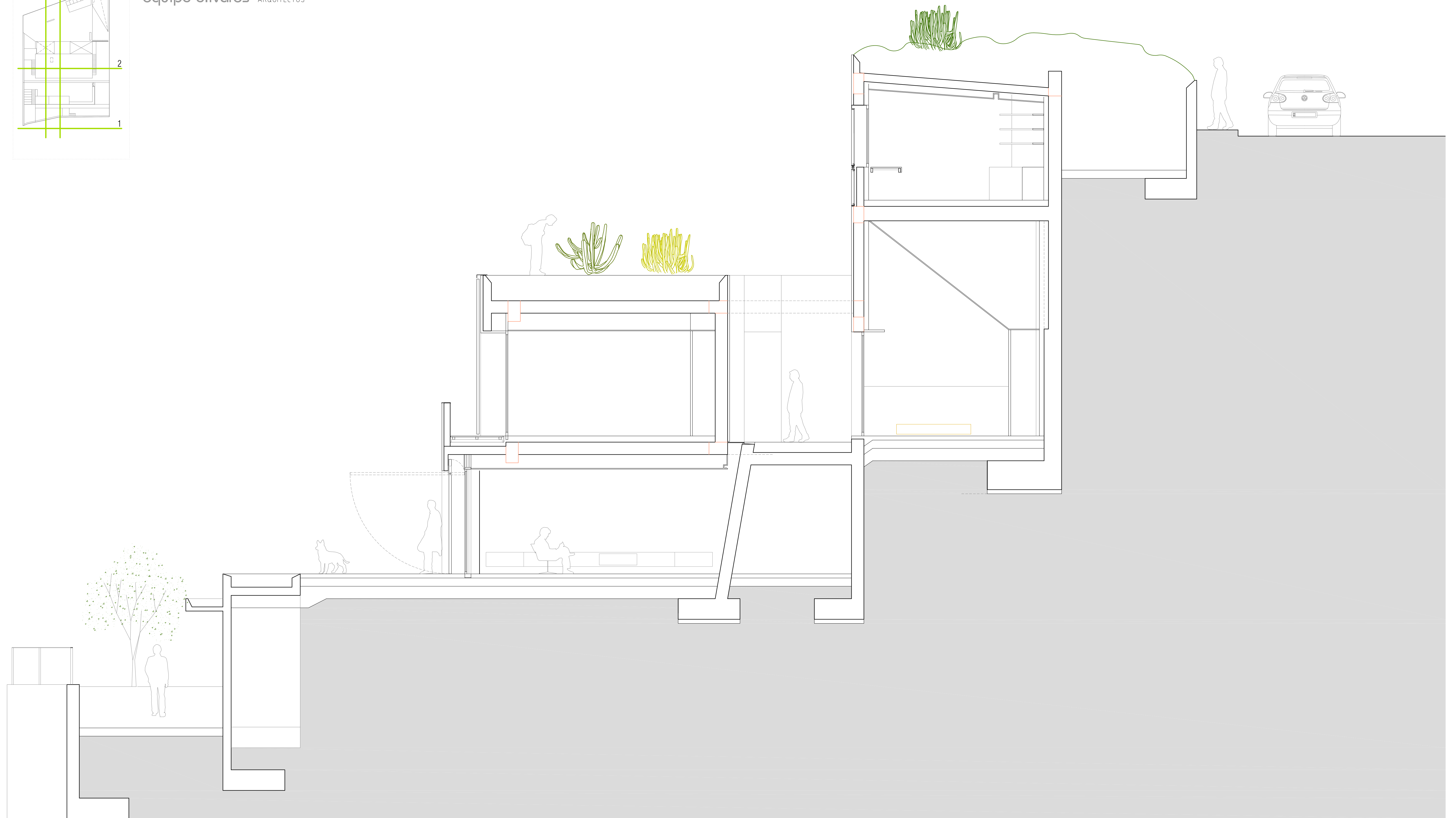
SECCIÓN LONGITUDINAL a
