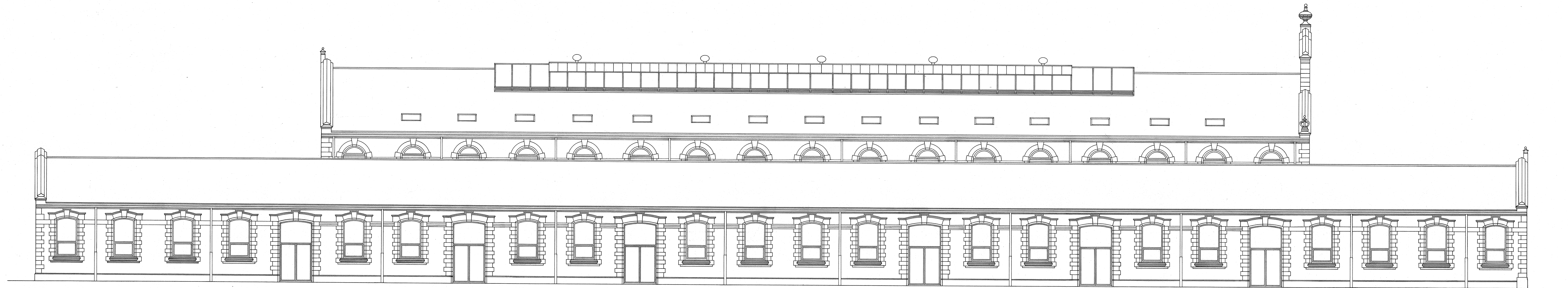
ALZADO 4
