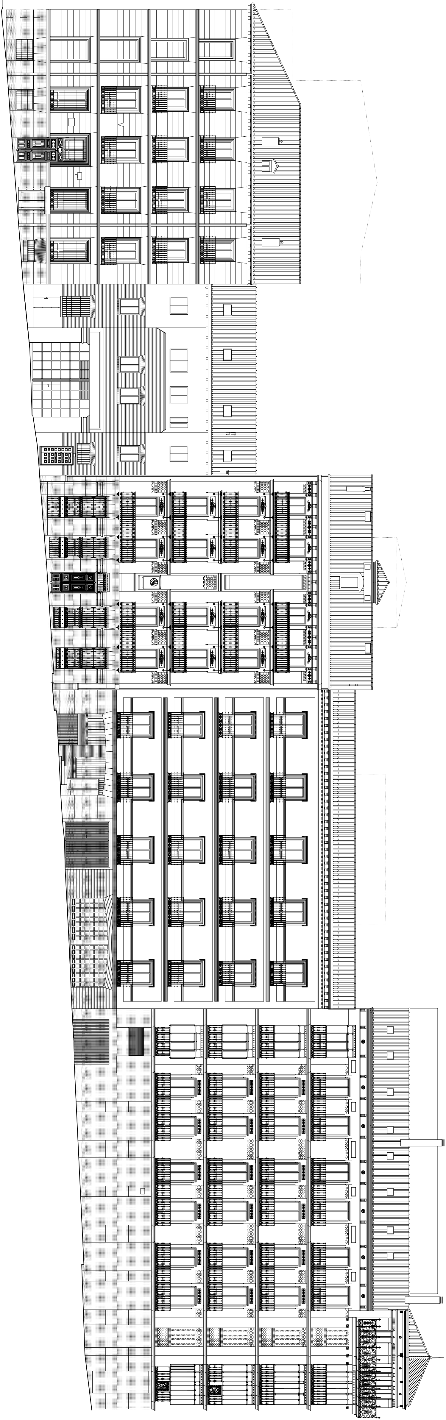
ALZADO ESTADO ACTUAL A LA CALLE CERVANTES
