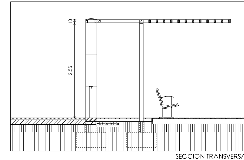
SECCION TRANSVERSAL
