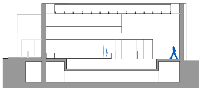
SECCIÓN C
