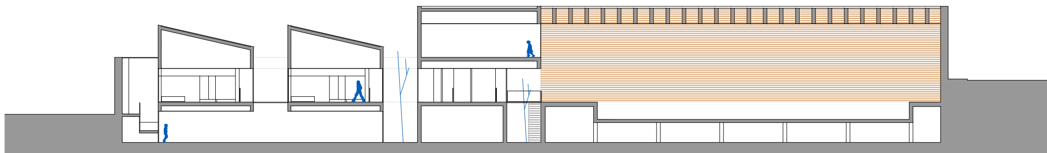
SECCIÓN B
