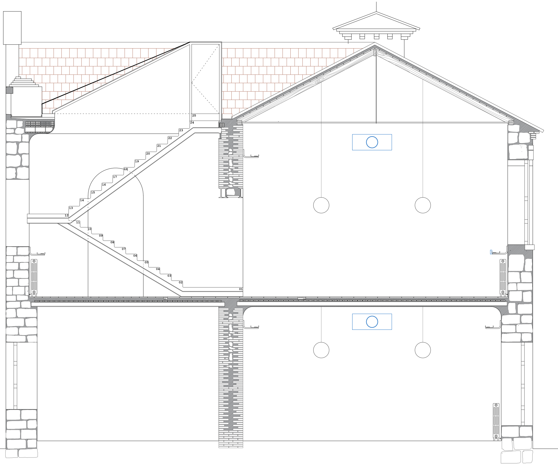
sección transversal. intervención
