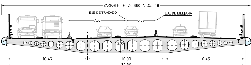
SECCION TRANSVERSAL TRAMO 10 ESCALA 1:300
