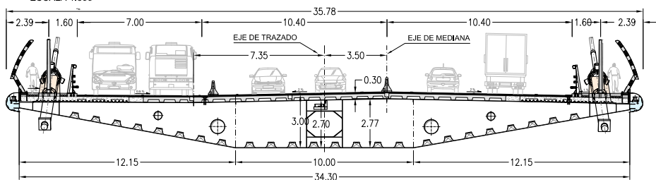
SECCION TRANSVERSAL TRAMO 6 ESCALA 1:300
