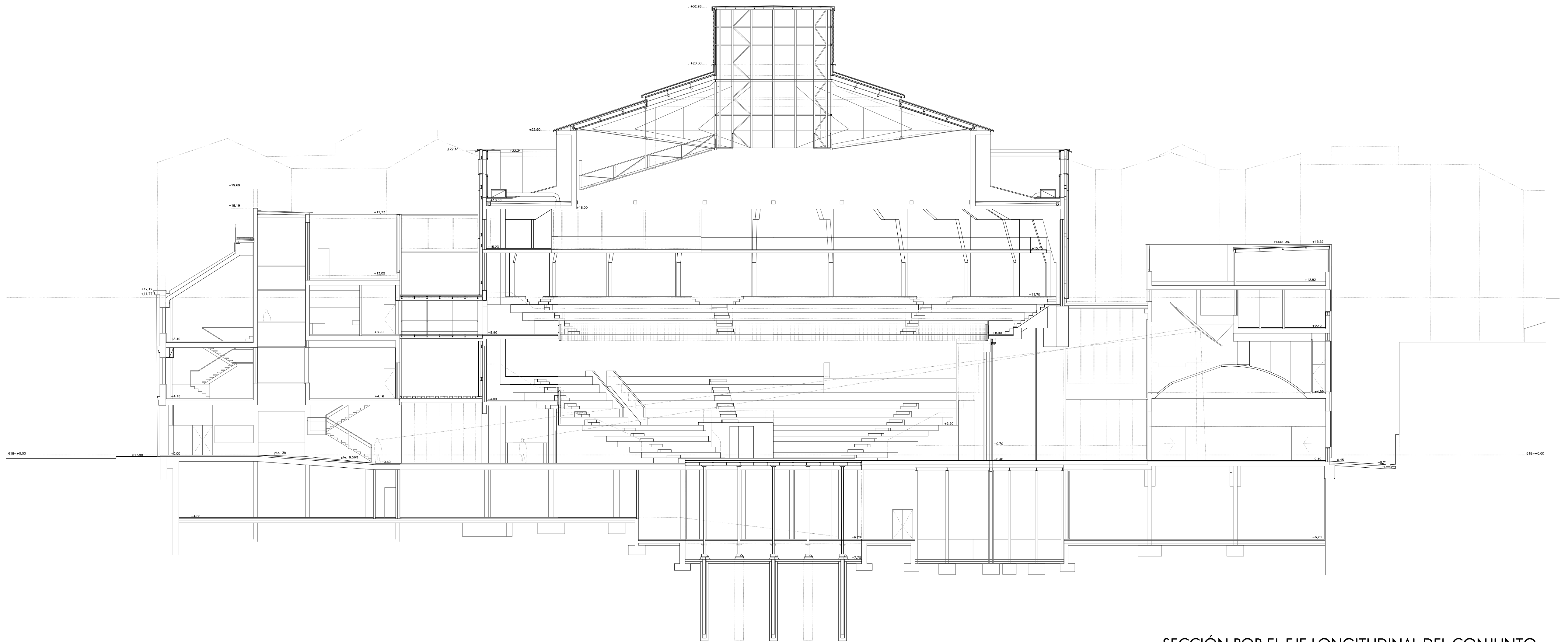
SECCIÓN POR EL EJE LONGITUDINAL DEL CONJUNTO
