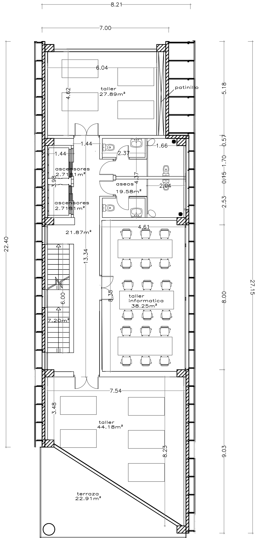
PLANTA SEGUNDA rasante +7,10
