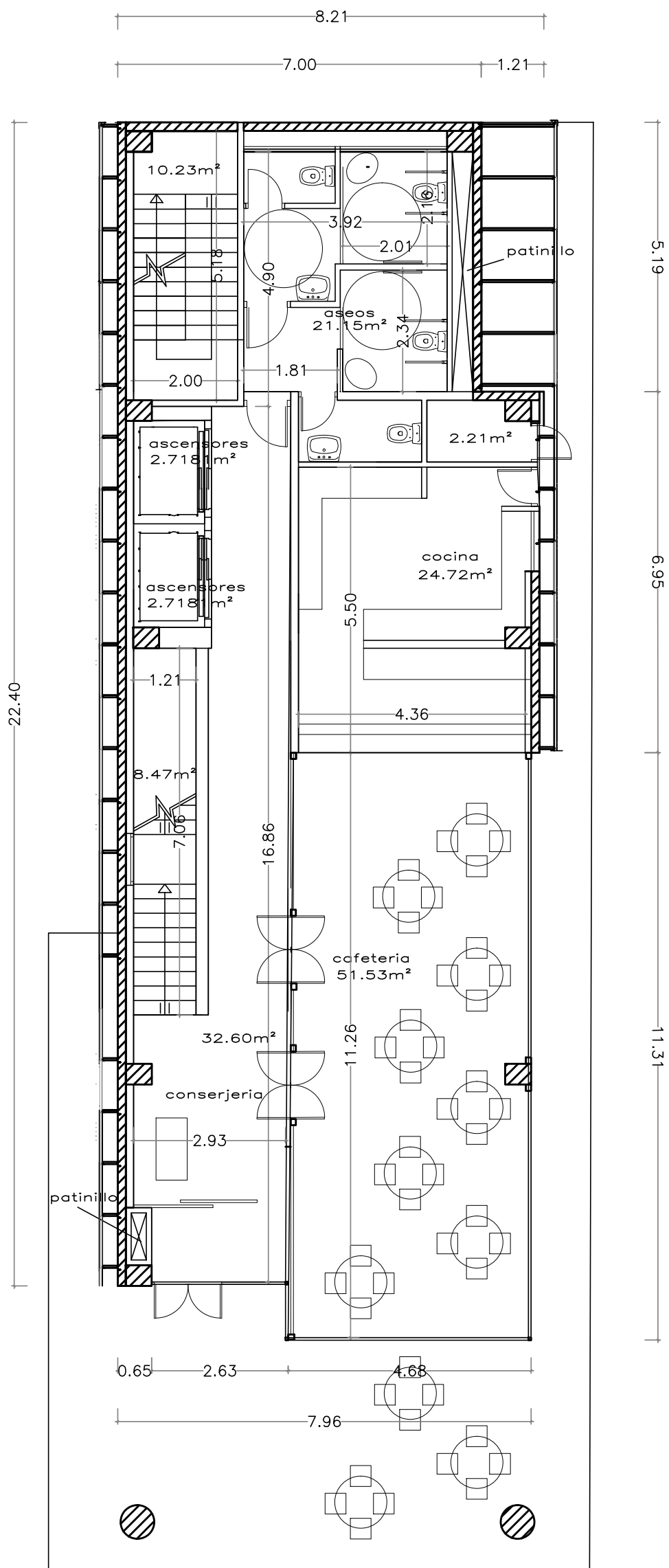
PLANTA BAJA rasante \pm 0,00
