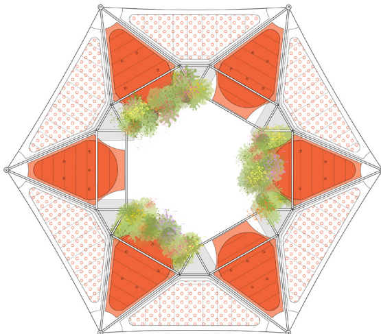
NIVEL DE CUBIERTA +14'-6 1/2" [4.43 m]
