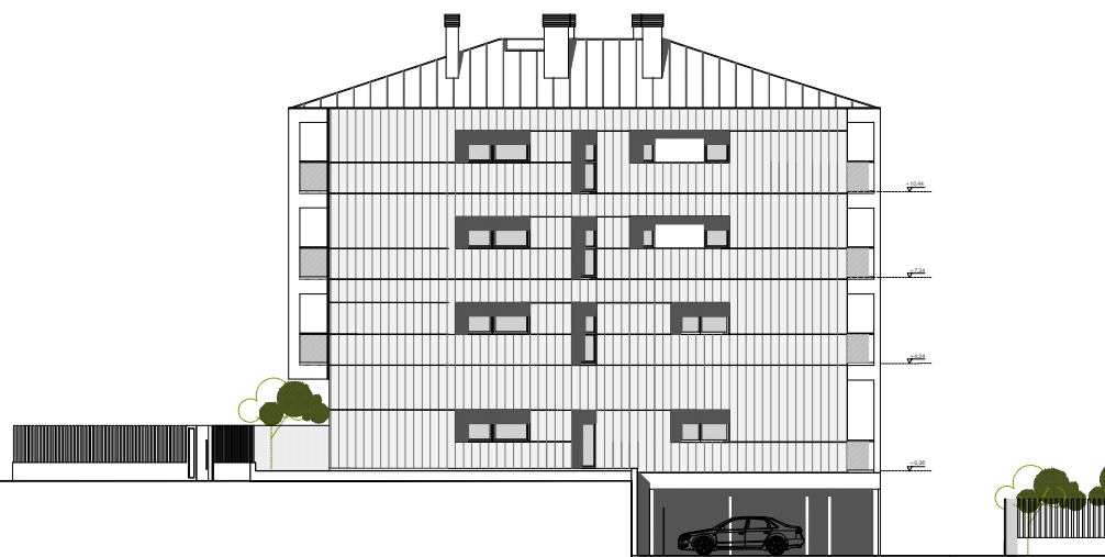
ER 05. Alzados y Sección longitudinal
