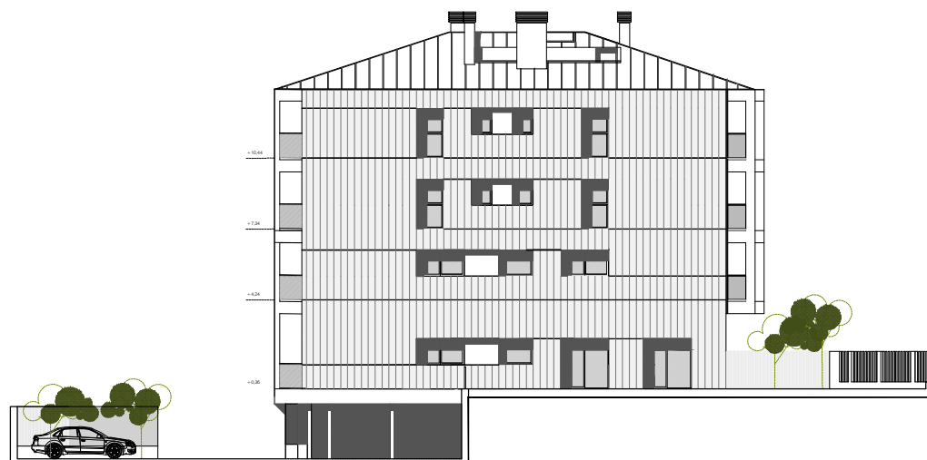
Alzados laterales
