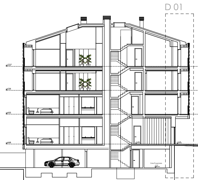
Sección longitudinal
