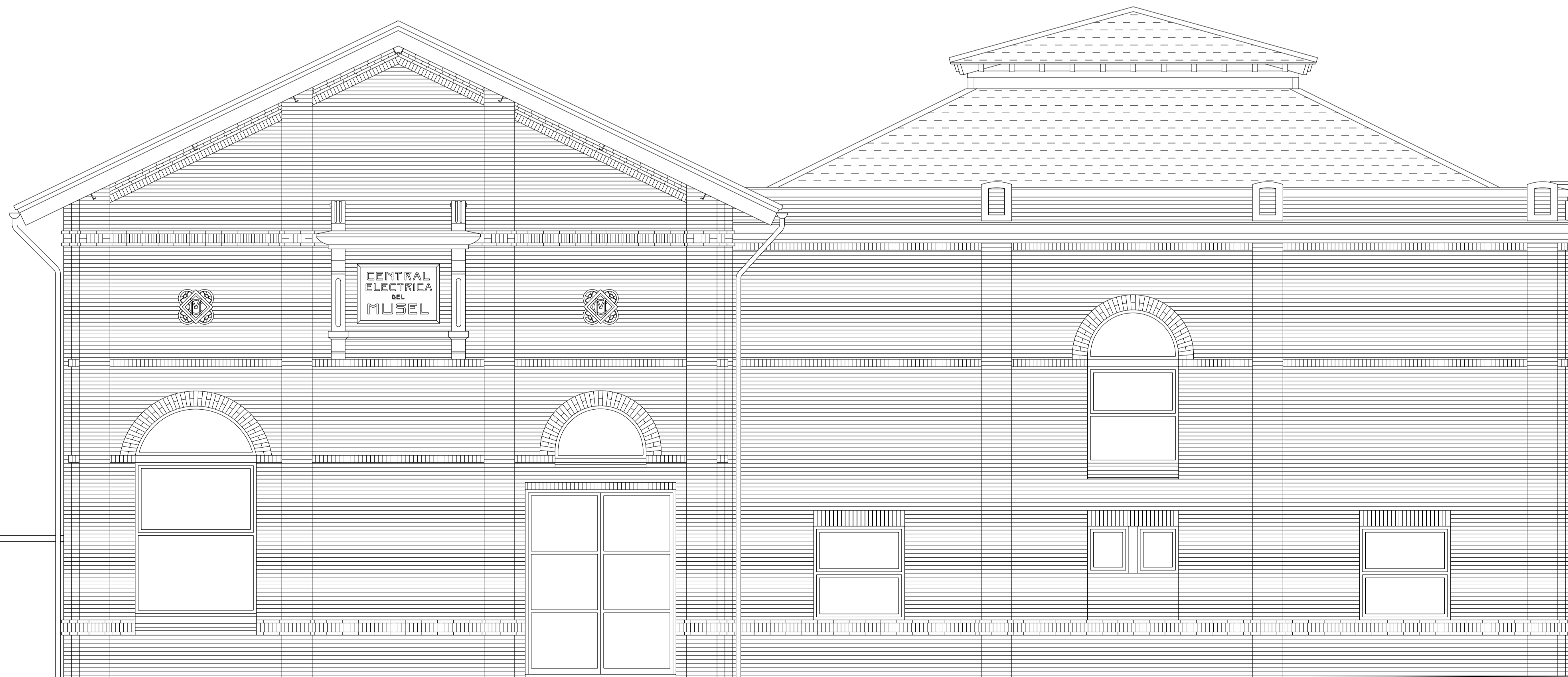
ALZADO NORTE
