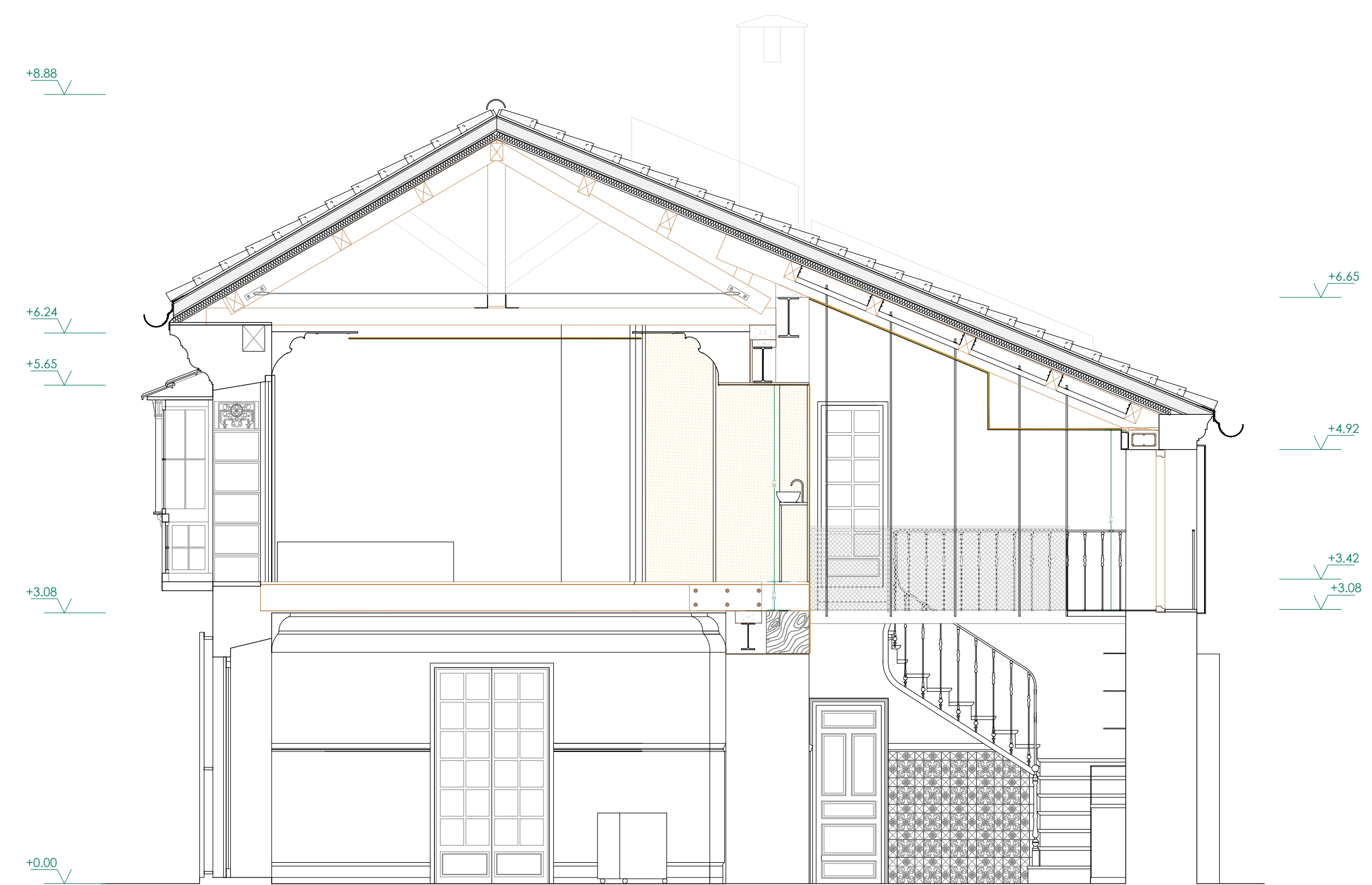
SECCIÓN B
