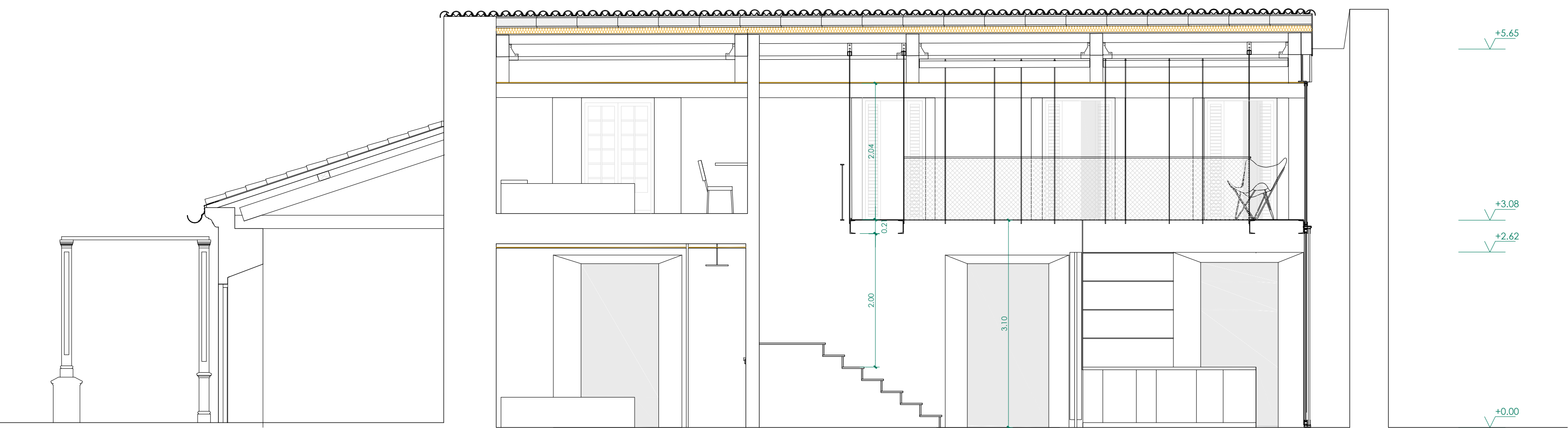
SECCIÓN A
