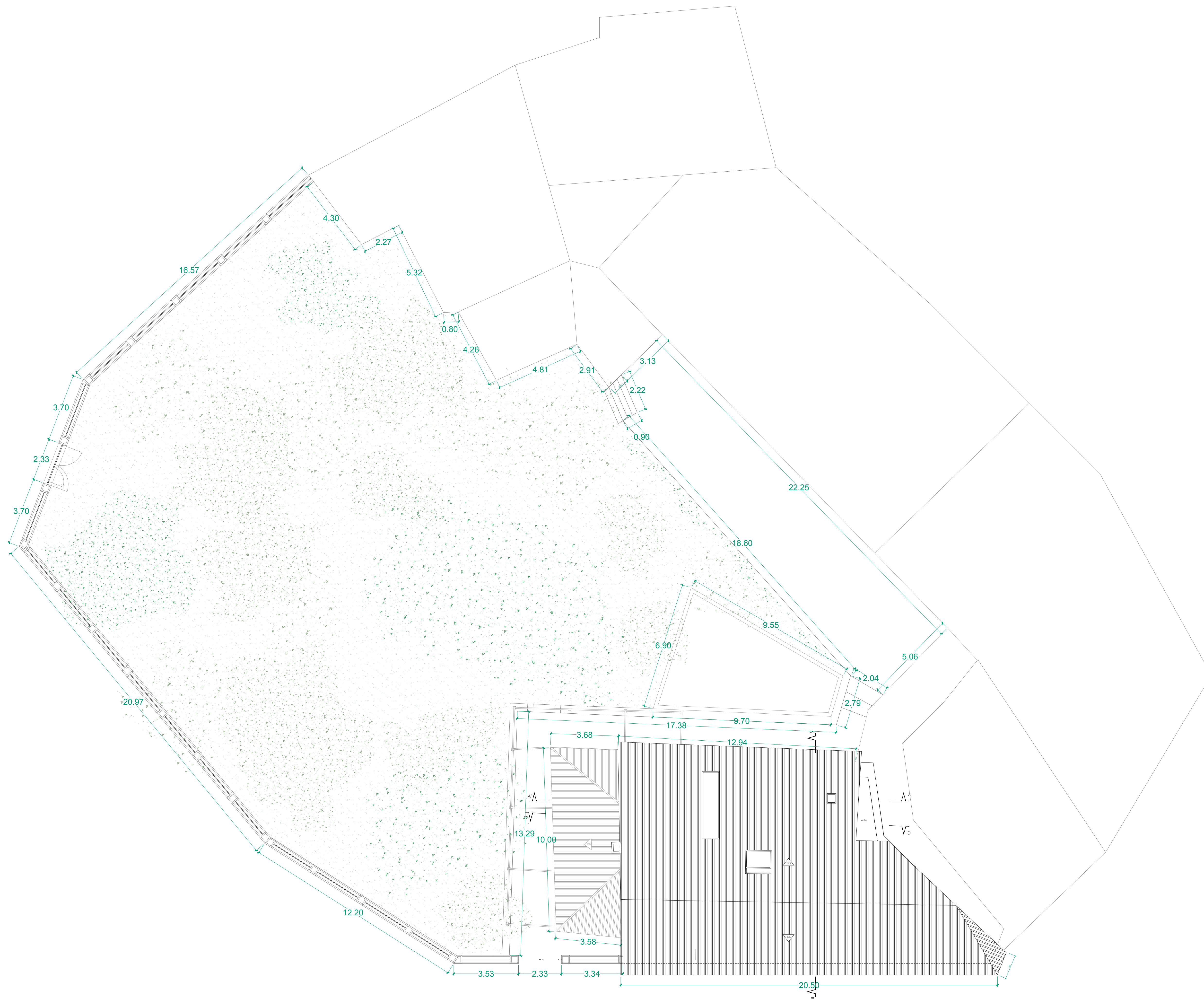
PLANTA DE CUBIERTAS
