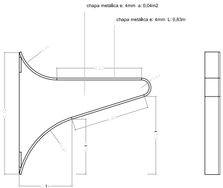
DETALLE BANCO
