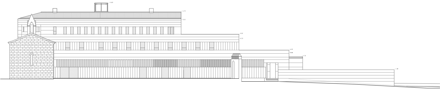
ALZADO ESTE
